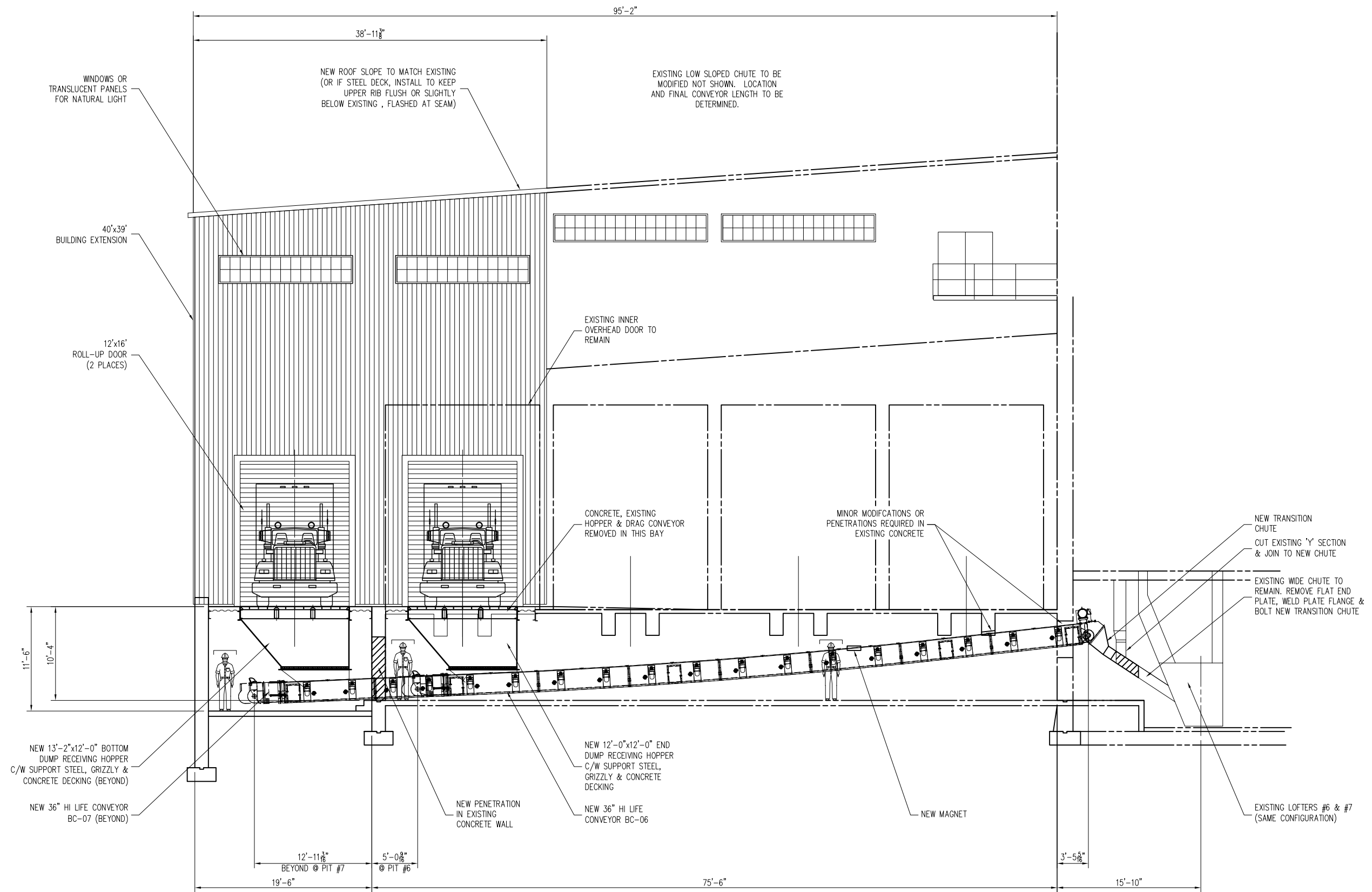
ELEVATION
