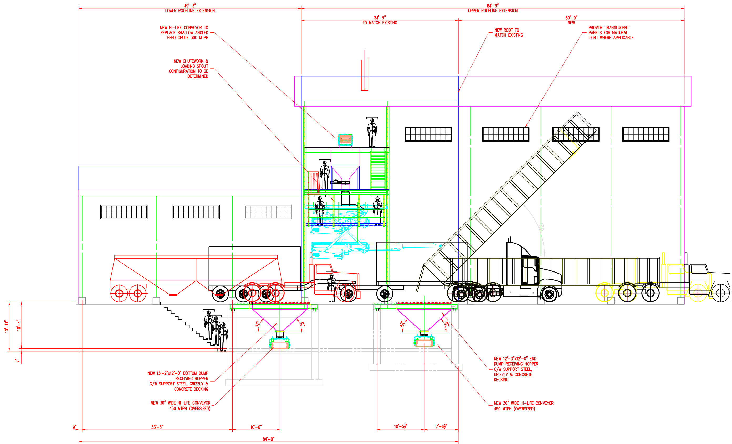
ELEVATION
